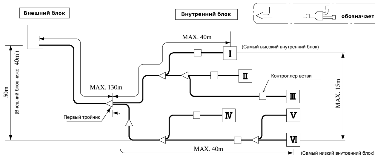
Допустимая длина трубопровода, перепад высот между внутренним и внешним блоками
