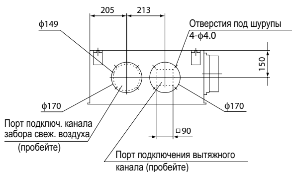
ВИД В
