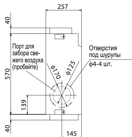
ВИД А
