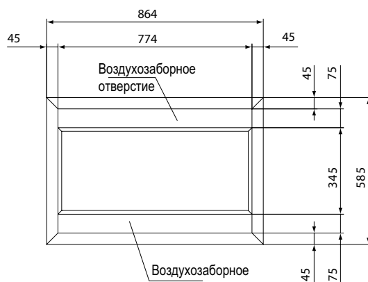
ВИД А
