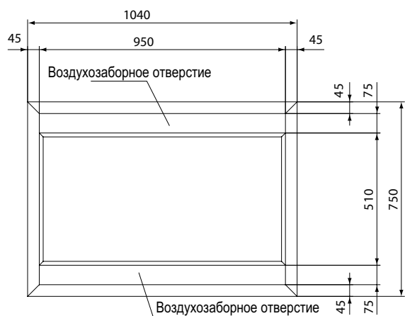
ВИД А
