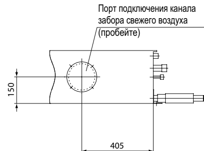
ВИД С
