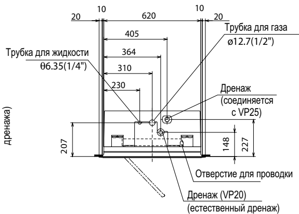
ВИД А
