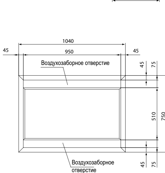
ВИД А
