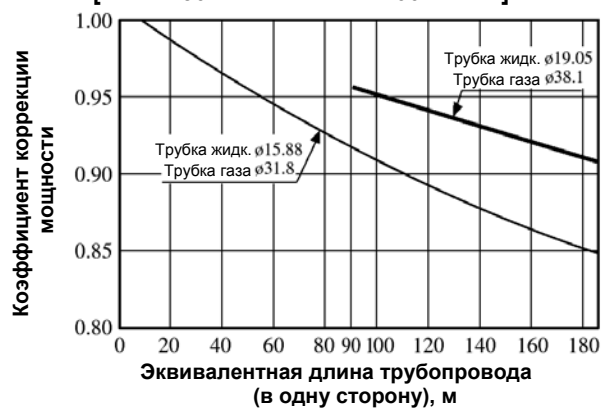
Модель FDCA900HKXE4 [FDCA450HKXE4 + FDCA400HKXE4]
